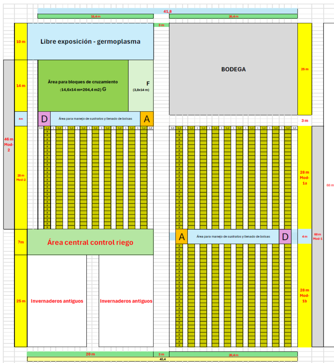
Figura 1. Esquema general de distribución de los invernaderos a construir y sus áreas anexas.
